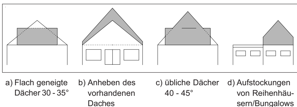
Abb. 4: Möglichkeiten des Dachausbaus bei Ein-/und Zweifamilienhäusern [3]
