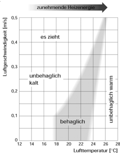
Bild 1: Behaglichkeitsdiagramm [1]
